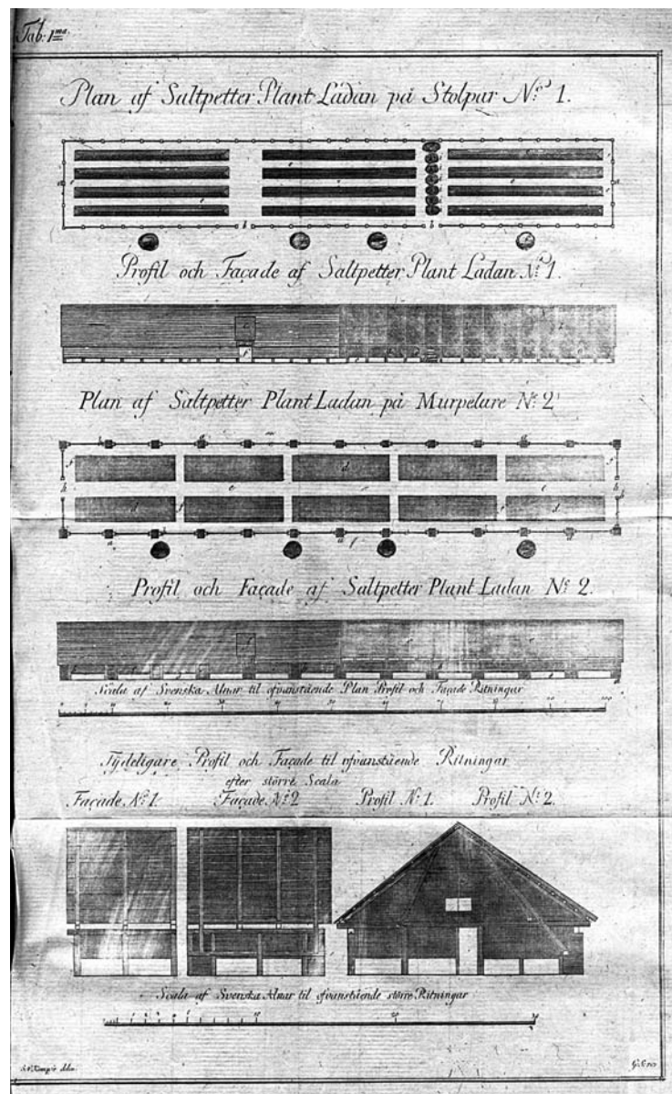
En principskiss över salpeterladornas konstruktion på 1700-talet.
